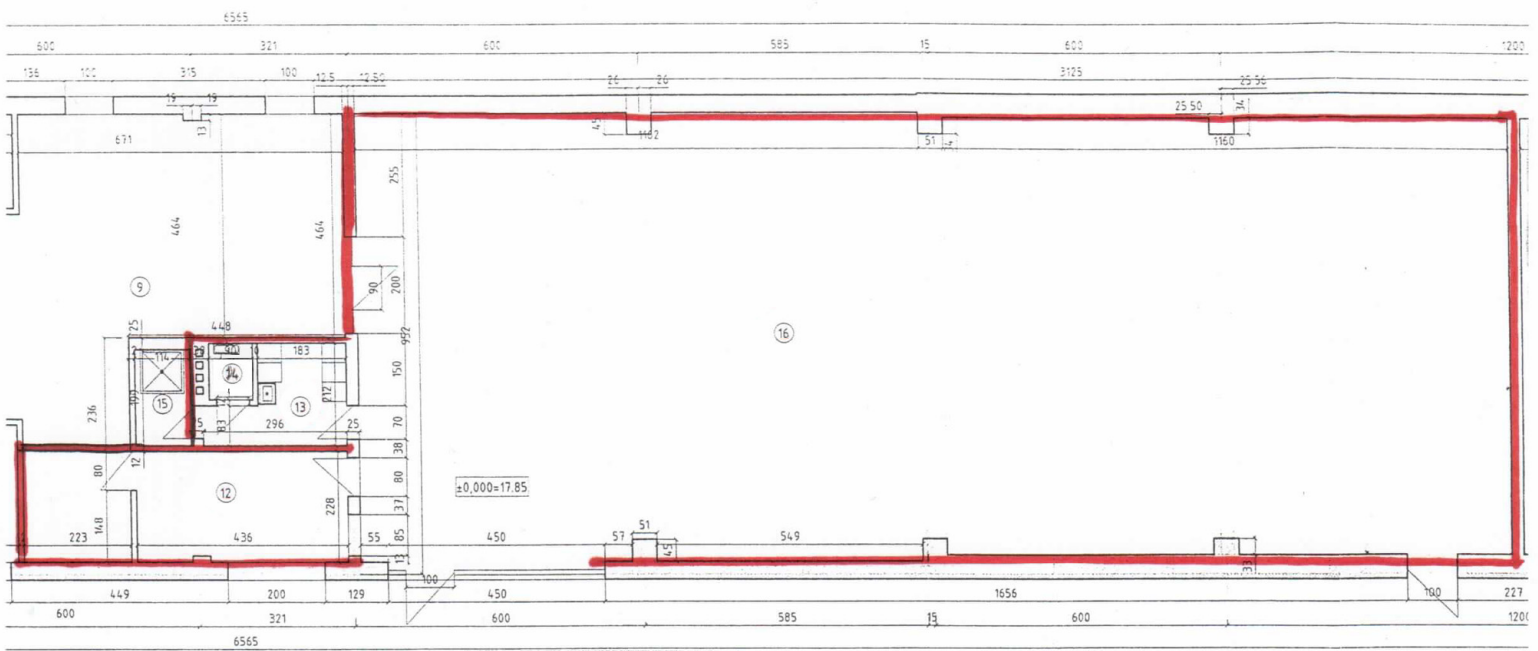
PIRMO AUKŠTO PLANAS
